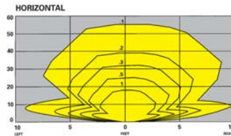
4 12 Volt, 9 Watt Tungsten Wedge Base
