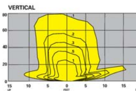
17 6 Volt, 8.0 Watt Tungsten Par 36
