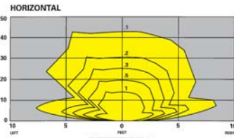
3 6 Volt, 9 Watt Tungsten Wedge Base PS
