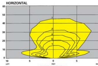
2 6 Volt, 7.2 Watt Tungsten Wedge Base PS
